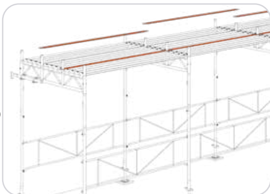
Spaltabdeckung für Passagenrahmen
